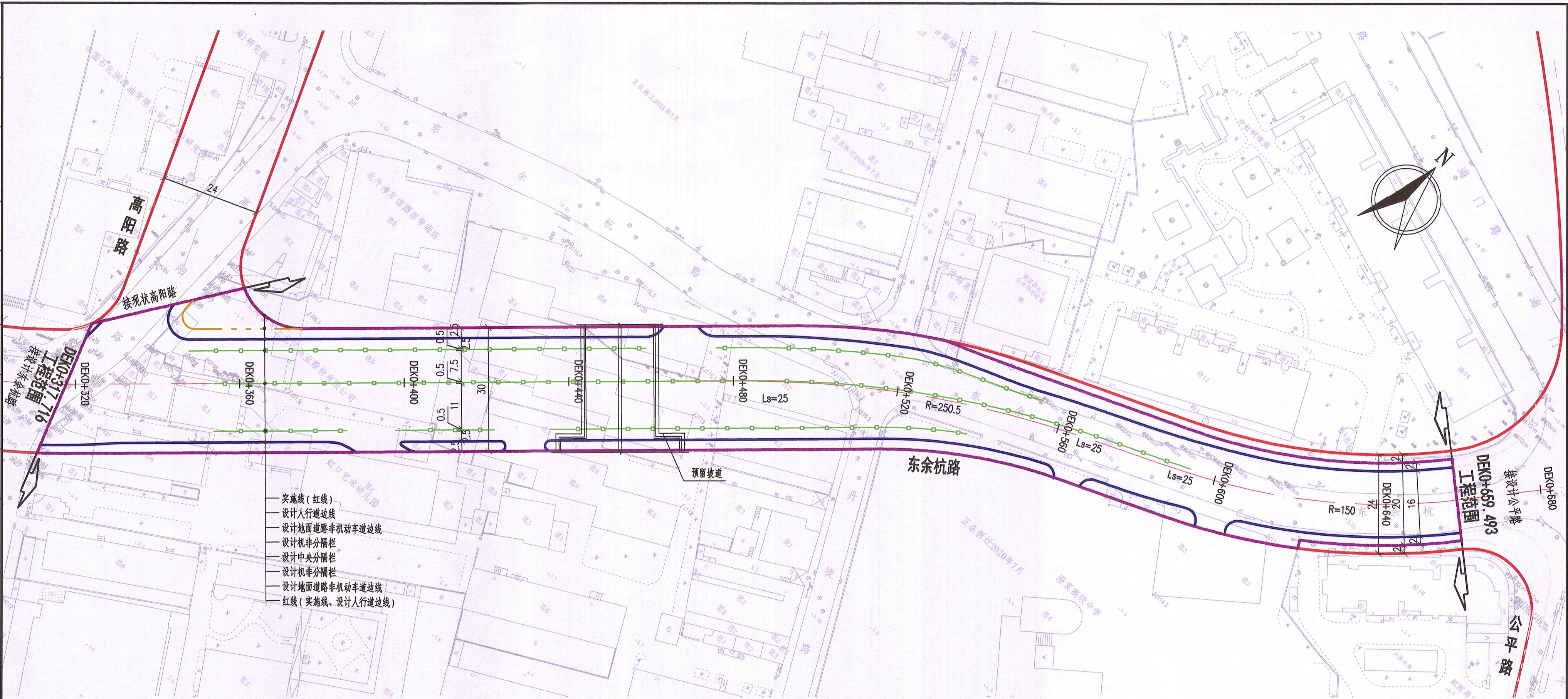
建设方案总平面公示图 (1:1000)
